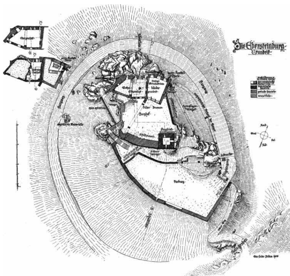
13. Burgruine Ebersteinburg, Grundriß
